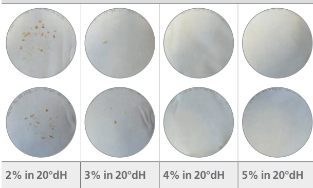
Test di corrosione del truciolo su carta DIN 51360/2 di Castrol Hysol SL 35 XBB
